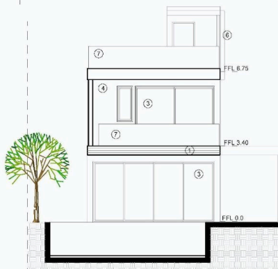
Οψη Α 1:100
