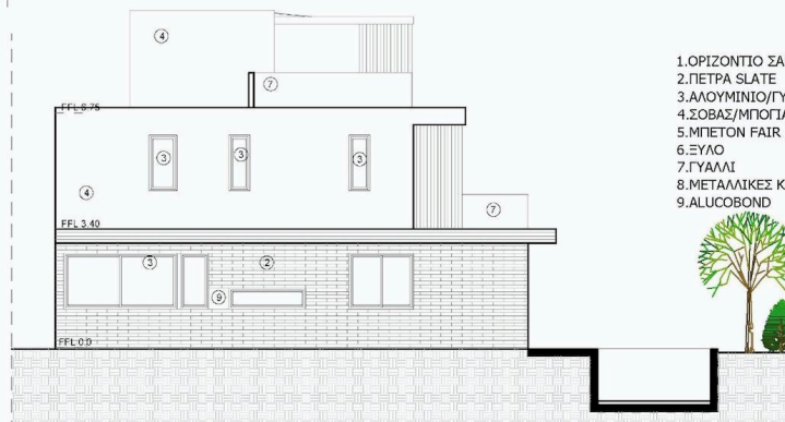
Οψη Β 1:100
