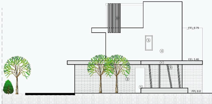
Οψη Β 1:100
