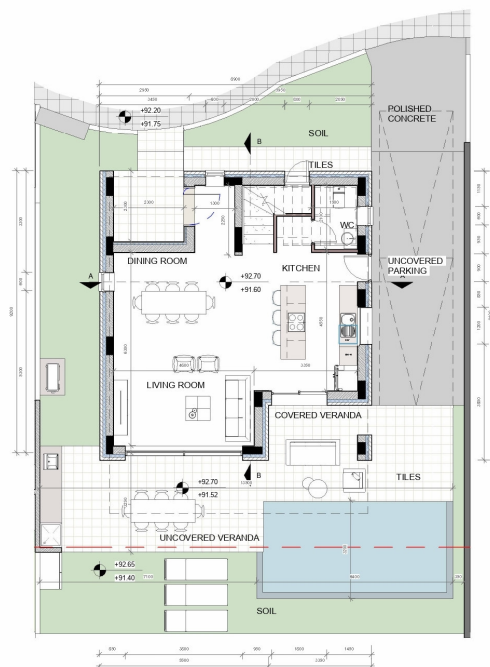
ΚΑΤΟΙΚΙΑ 12 ΚΛΙΜΑΚΑ 1:100 ΕΜΒΑΔΟΝ = 64.70 τ.μ.
