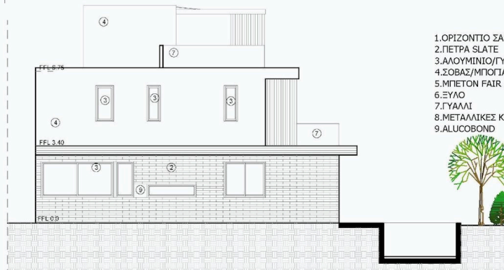
ΟΨΗ Β 1:100
