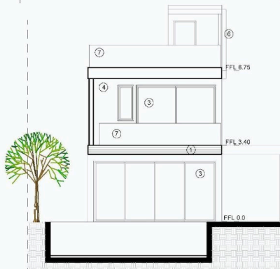
ΟΨΗ Α 1:100
