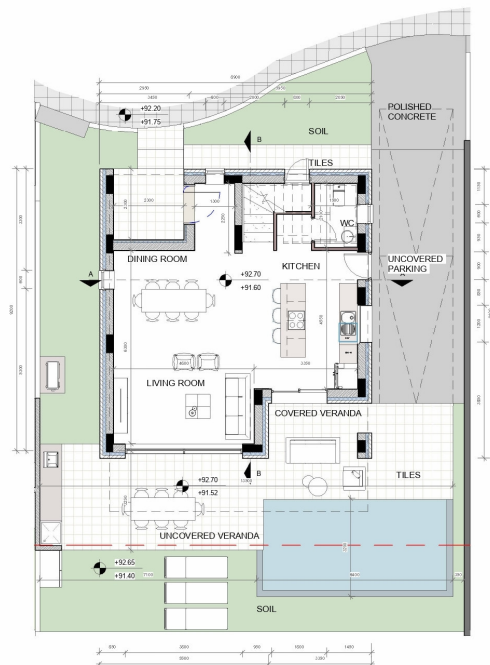
ΚΑΤΟΙΚΙΑ 12 ΚΑΙΜΑΚΑ 1:100 ΕΜΒΑΔΟΝ = 64.70 τ.μ.
